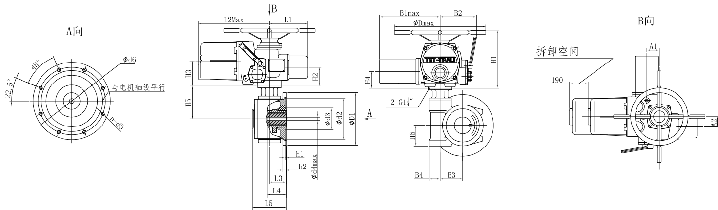
SMC-04~03带HBC外形及连接尺寸
